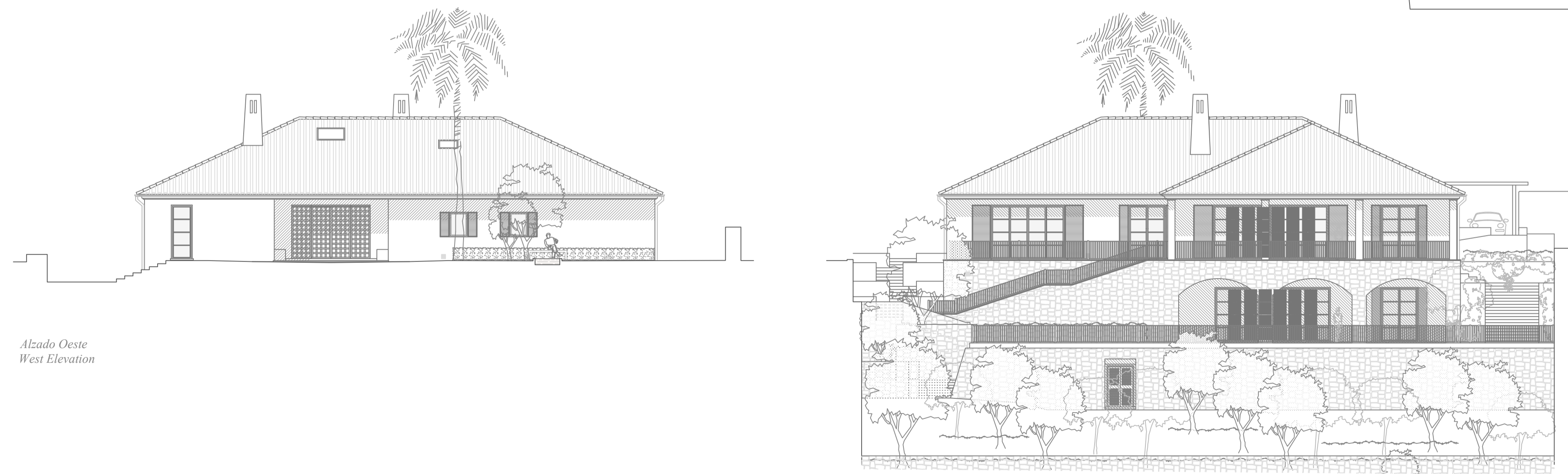
Alzado Este East Elevation
