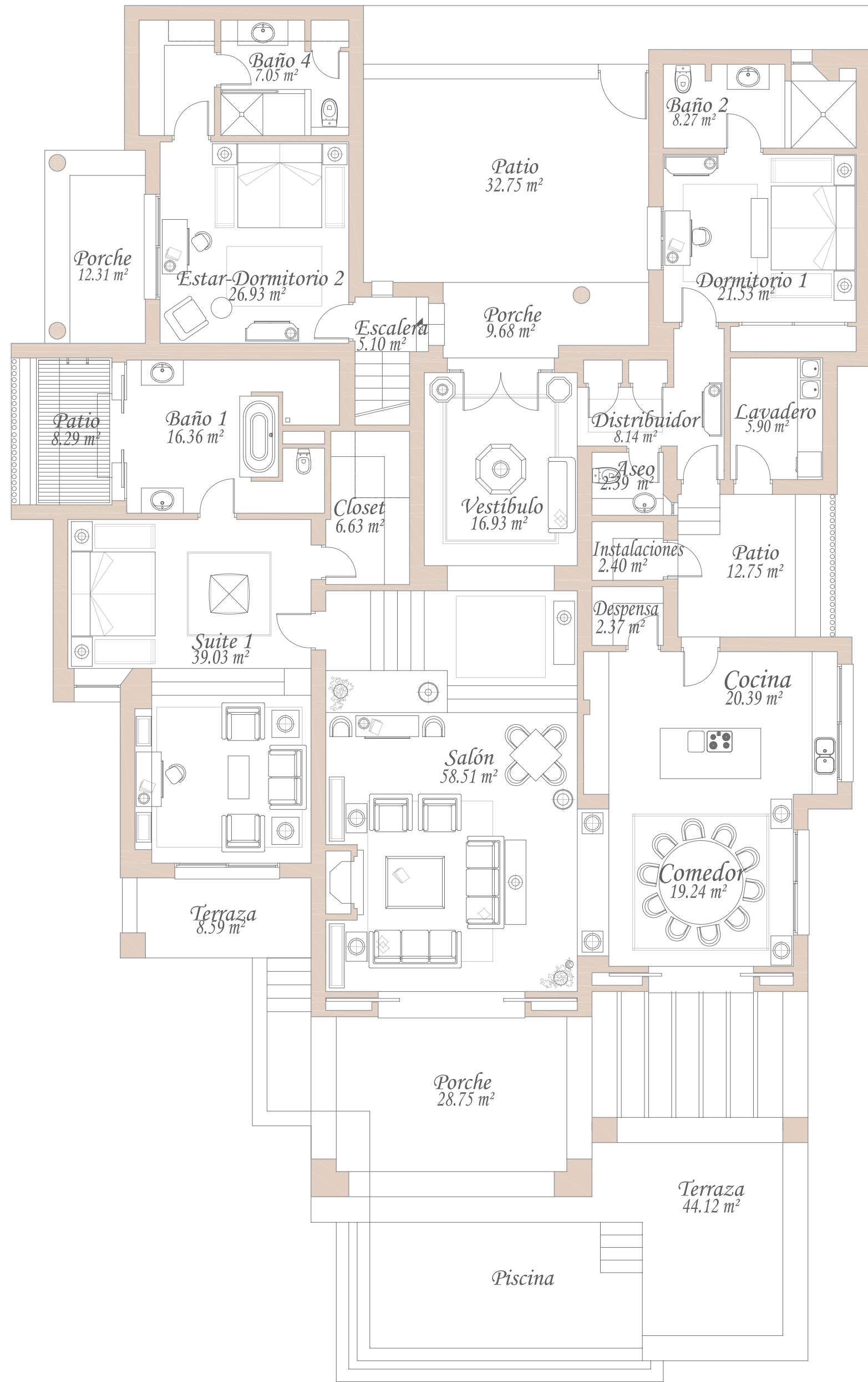
Planta Baja
