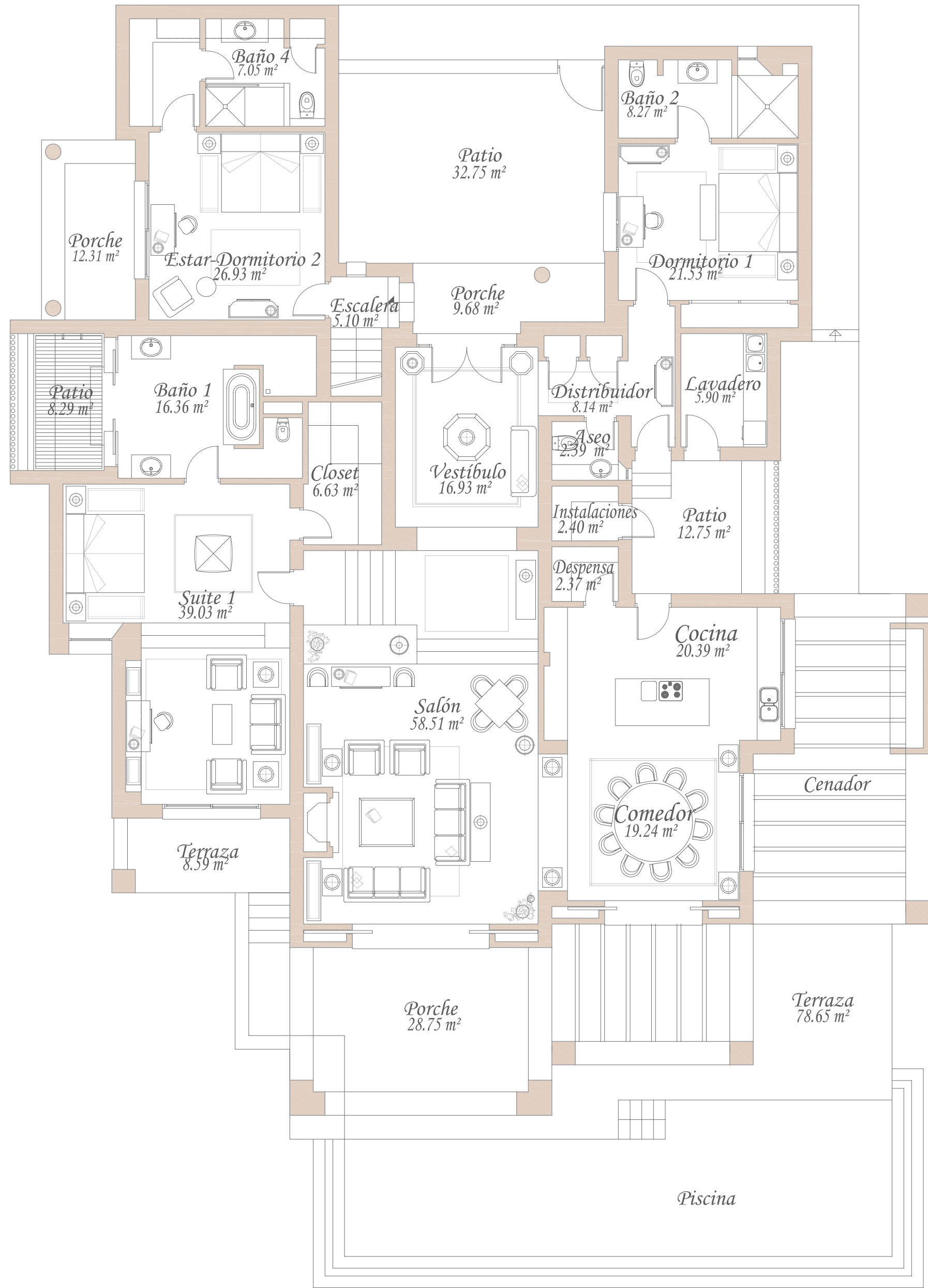
Planta Baja
